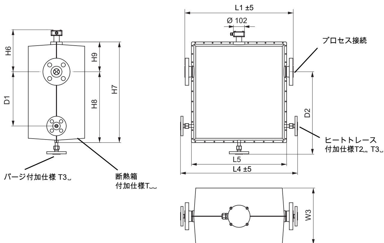
図 21: 寸法 (単位 mm):断熱箱付き
