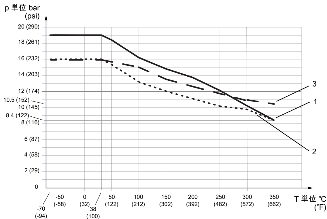
図 8: プロセス接続部の温度と許容プロセス圧力の関係
