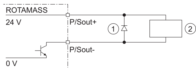
図 30: アクティブパルス出力接続 P/Sout の機械式カウンタとの接続図
