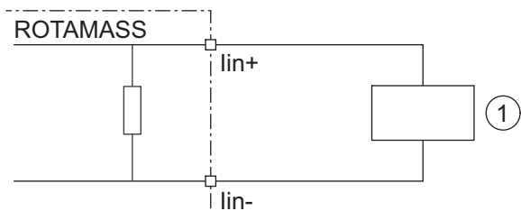
図 28: アクティブ電流出力をもつ外部機器との接続図
