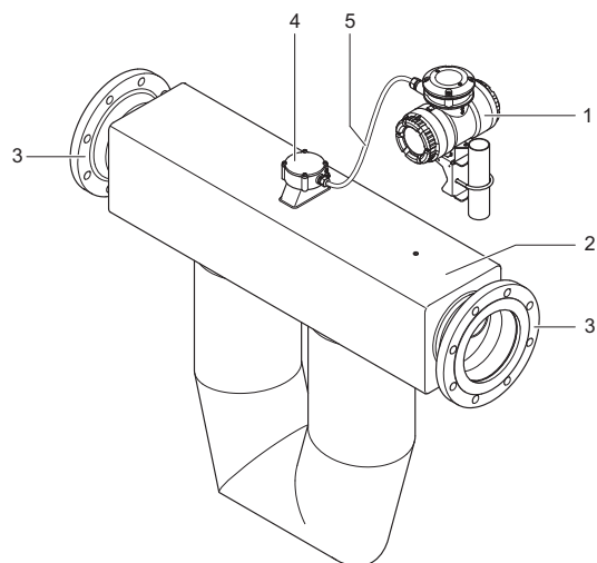
図 3: Rotamass 分離形の構造
