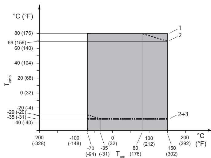
図 14: 許容される流体温度および周囲温度 (分離形)
