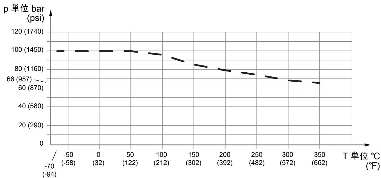
図 11: 流体温度と許容プロセス圧力の関係 (EN 1092-1 PN100 準拠フランジ)
