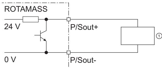
図 31: 内部プルアップ抵抗付き アクティブパルス出力 P/Sout
