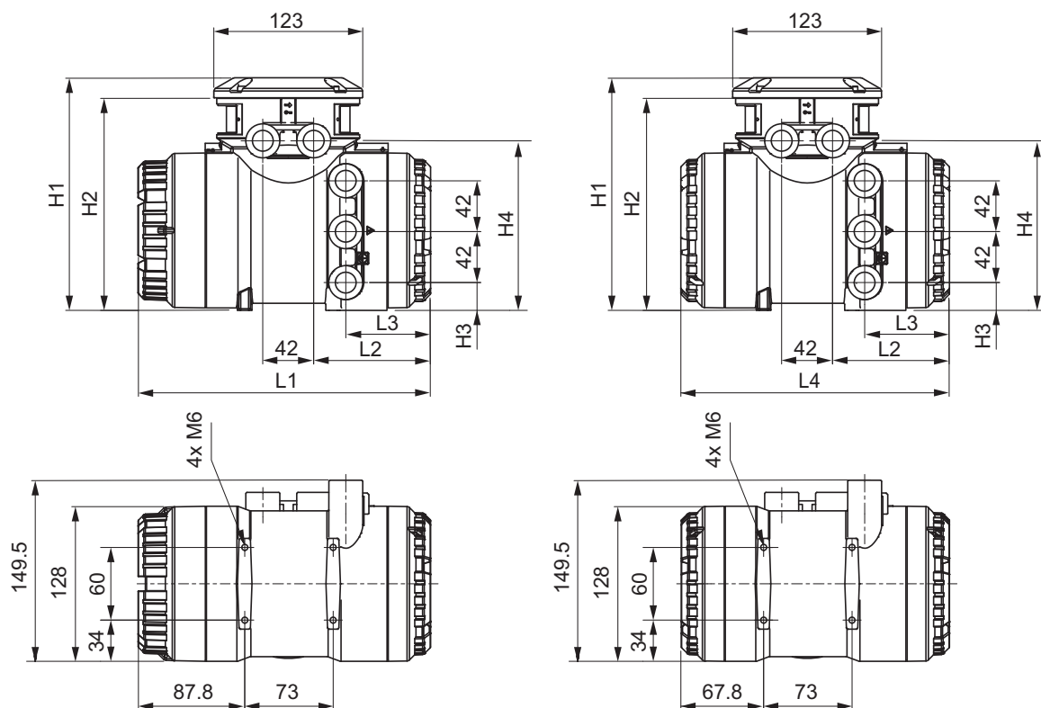
図 22: 変換器の寸法, 単位 mm, (左側: 表示器付き変換器, 右側: 表示器のない変換器)
