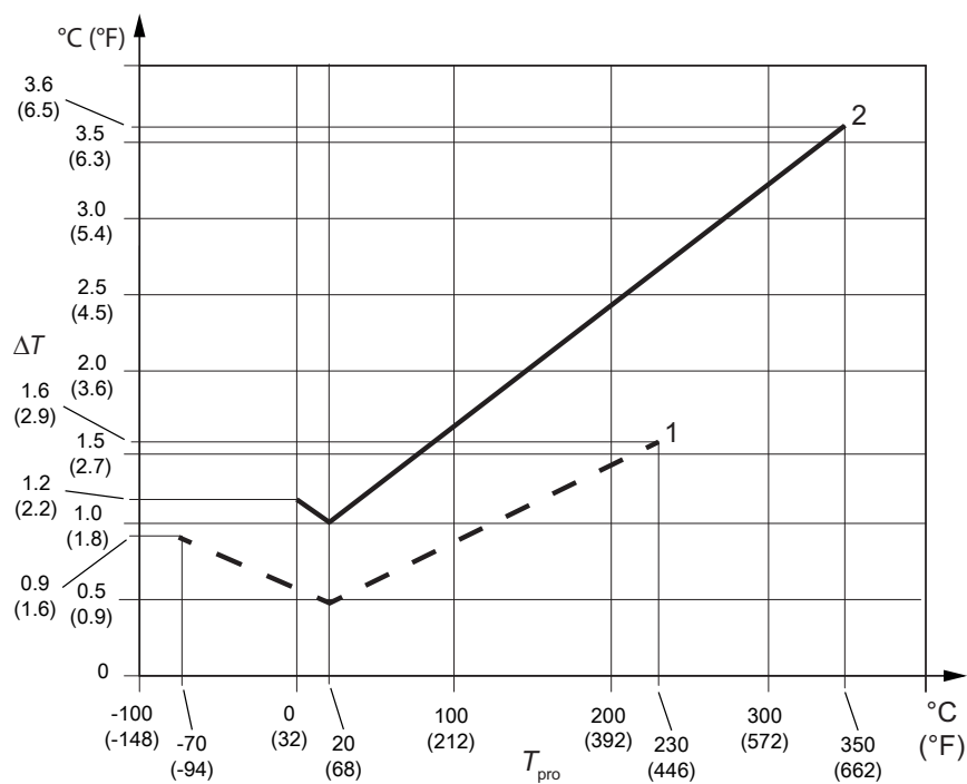
図 6: 温度の精度
