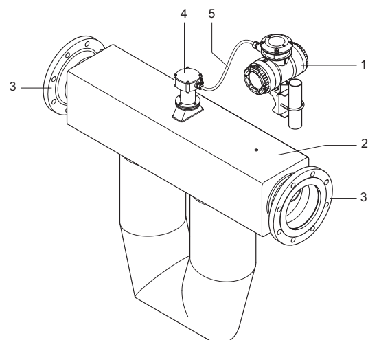
図 4: Rotamass 端子箱距離延長形の分離形の構造
