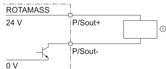
図 34: アクティブステータス出力接続 P/Sout
