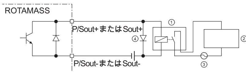
図 37: ソレノイドバルブ回路がある場合のパッシブステータス出力接続 P/Sout または Sout の接続図
