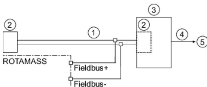
図 40: PROFIBUS PA 接続
