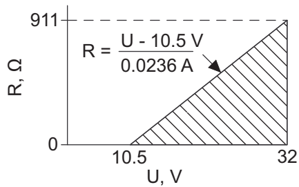
図 25: 外部電源電圧と最大負荷抵抗の関係
