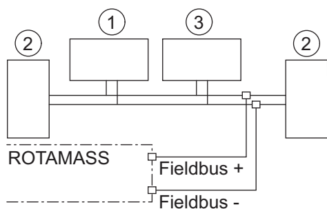
図 41: FOUNDATION Fieldbus 接続図
