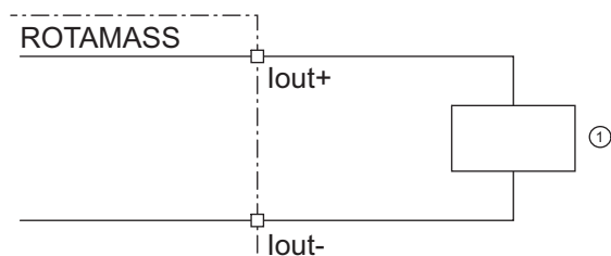
図 24: アクティブ電流出力接続 lout HART の接続図
