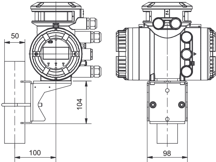
図 23: 変換器の寸法, 単位 mm, (U字金具に取り付け)
