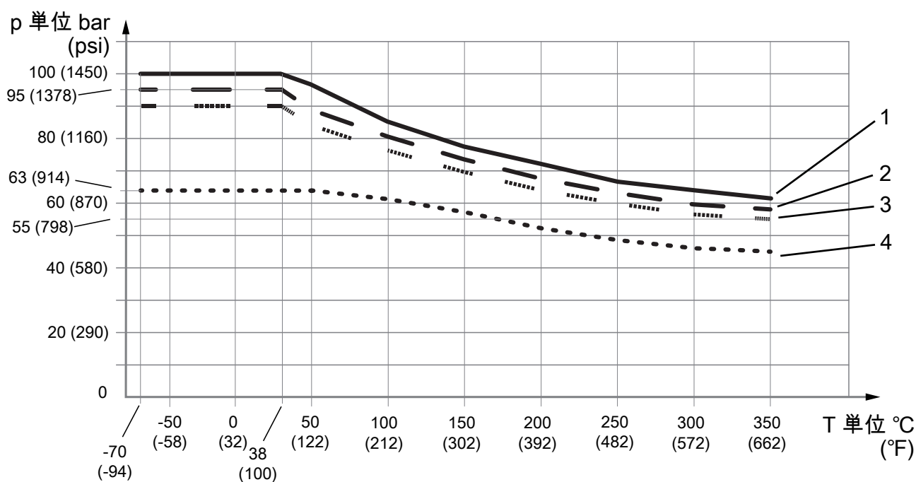
図 10: プロセス接続部の温度と許容プロセス圧力の関係
