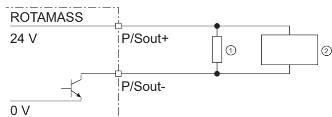
図 29: アクティブパルス出力接続 P/Sout の接続図
