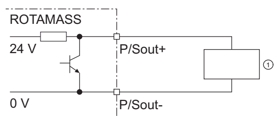
図 35: 内部プルアップ抵抗付き アクティブステータス出力 P/Sout
