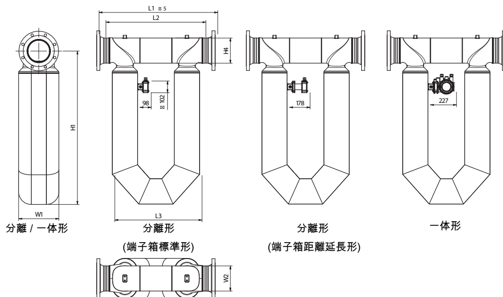
図 19: 寸法 (単位 mm)
