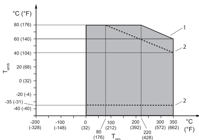
図 16: 許容される流体温度および周囲温度 (分離形)
