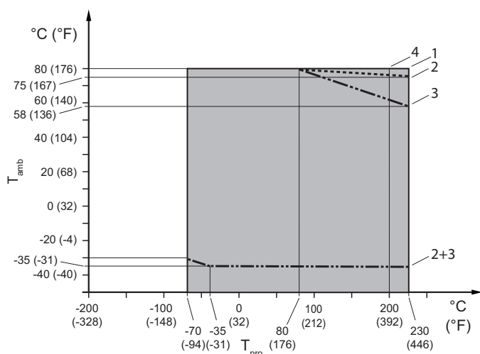
図 15: 許容される流体温度および周囲温度 (分離形)
