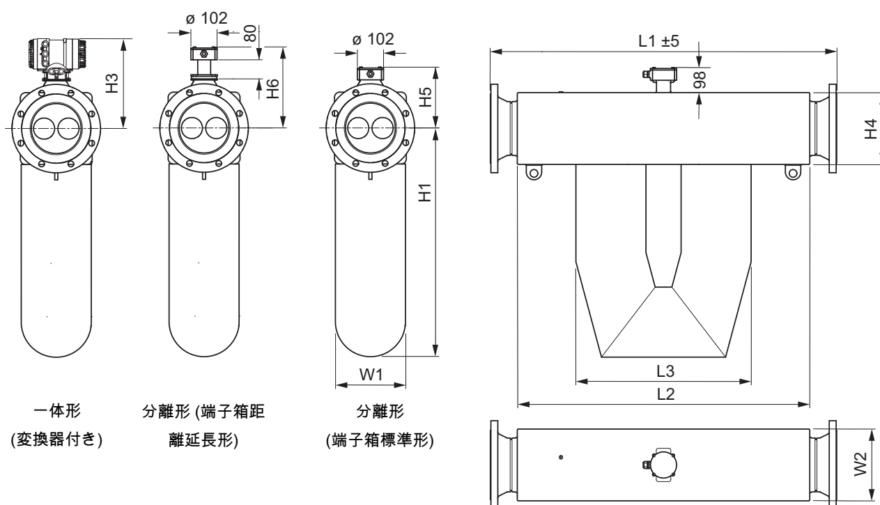
図 19: 寸法 (単位 mm)
