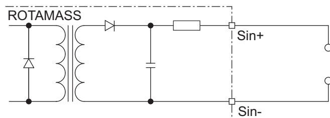
図 39: ステータス入力接続図
