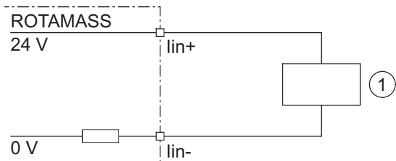
図 27: パッシブ電流出力をもつ外部機器との接続図
