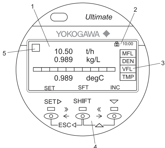
図 42: 表示器のレイアウト
