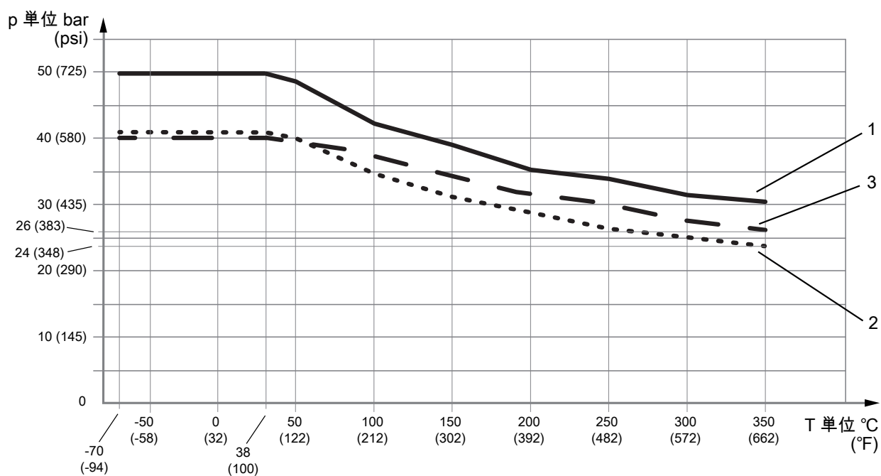
図 9: プロセス接続部の温度と許容プロセス圧力の関係
