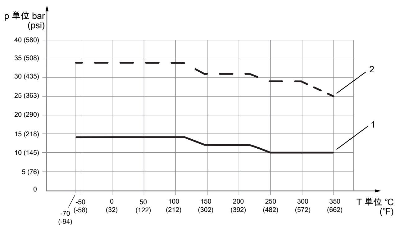
図 12: 流体温度と許容プロセス圧力の関係
