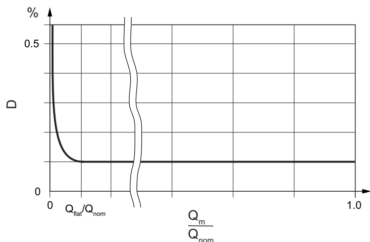
図 5:精度と質量流量の関係のグラフ
